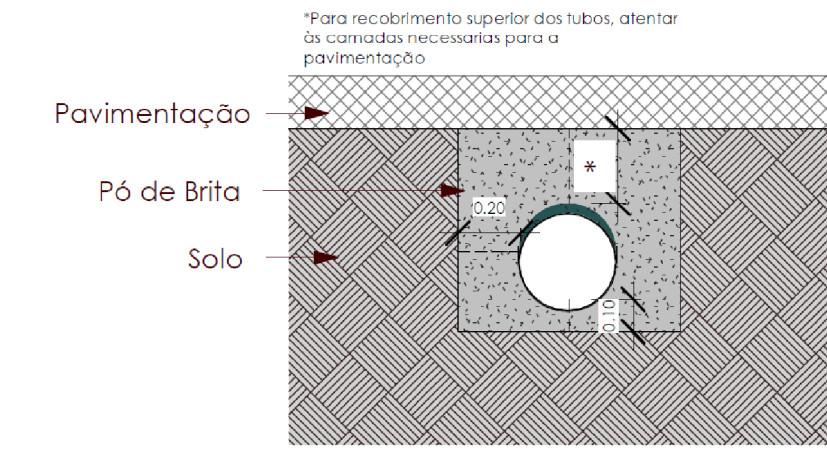
Detalhe execução da rede quando abaixo da pavimentação
